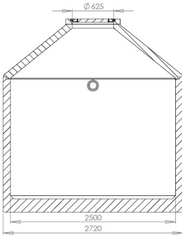
SCHNITT B-B
