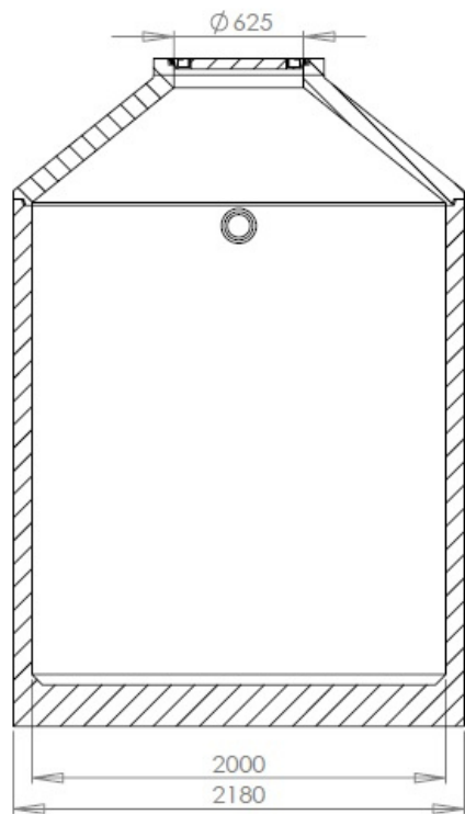
SCHNITT B-B
