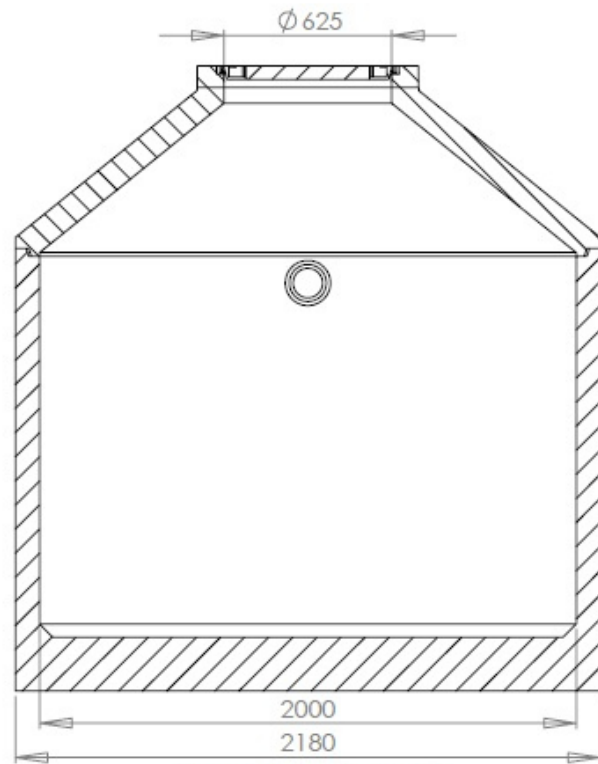
SCHNITT B-B
