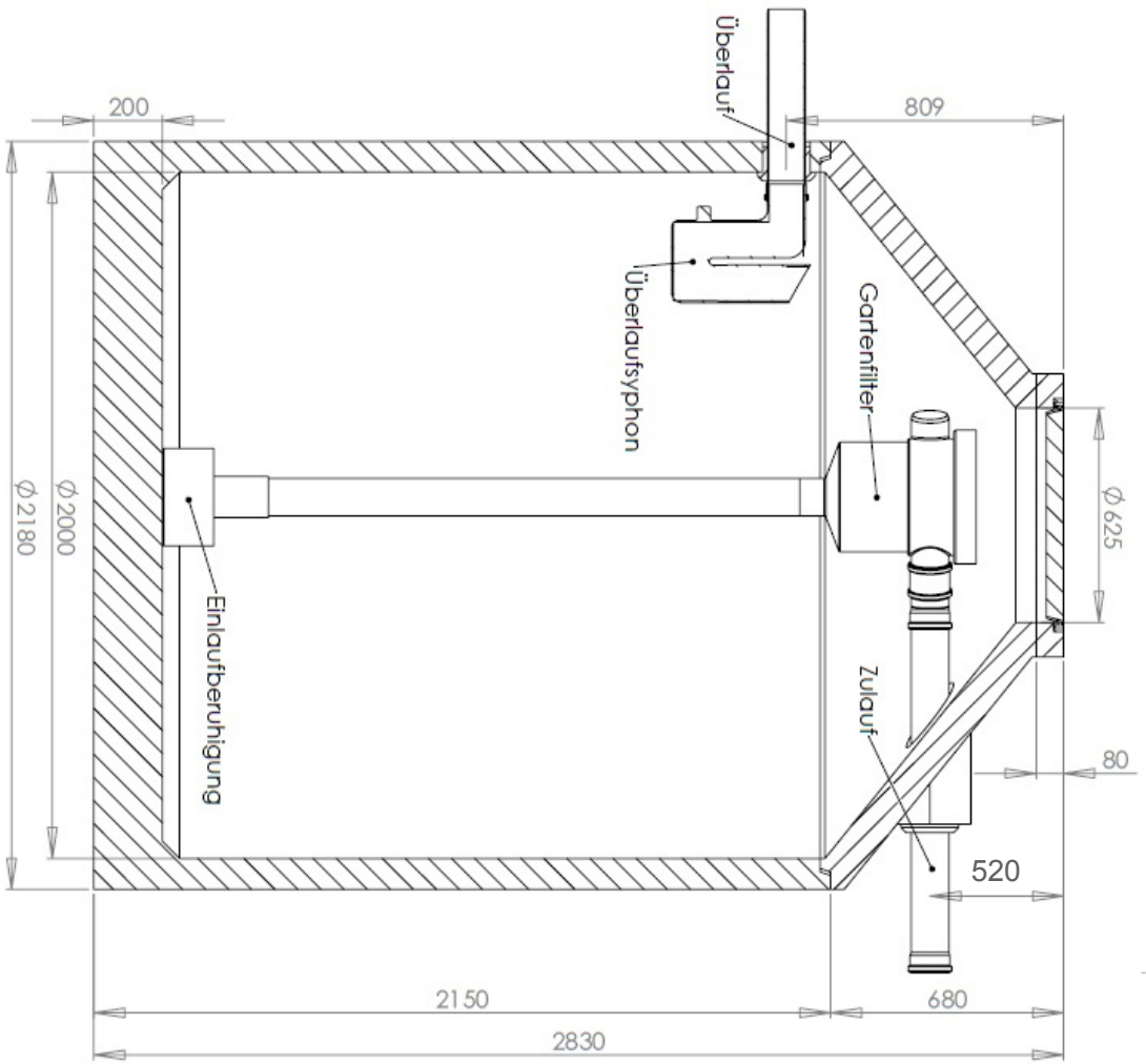
SCHNITT A-A
