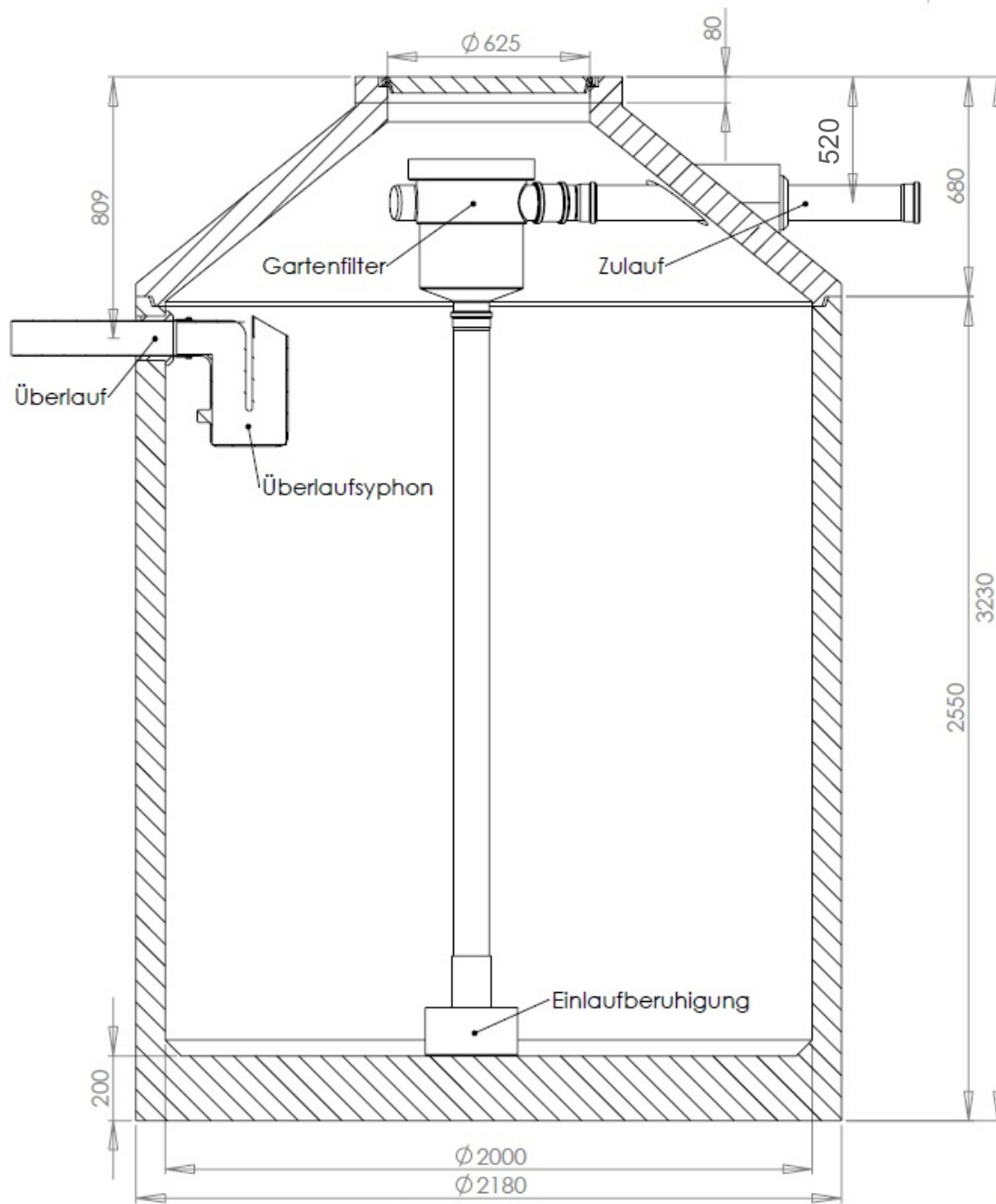
SCHNITT A-A
