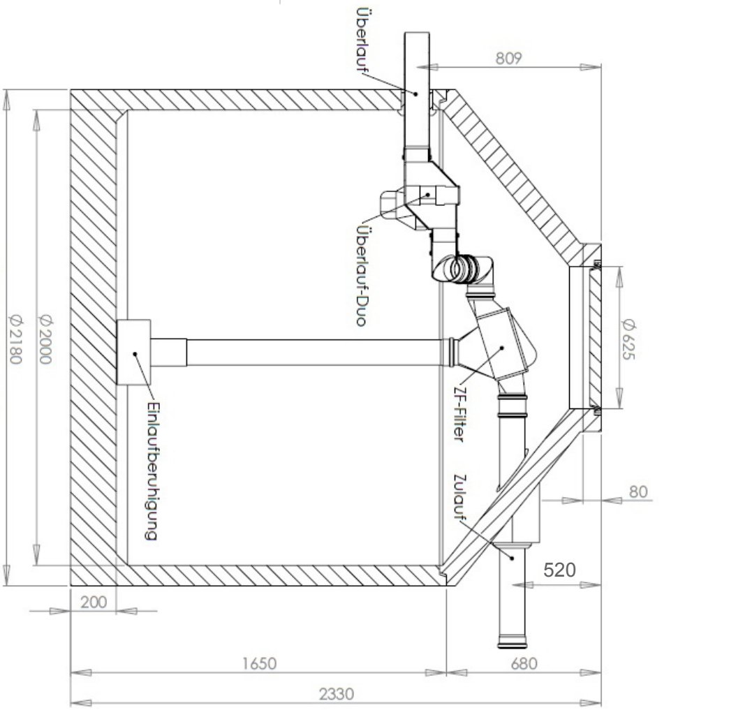
SCHNITT A-A
