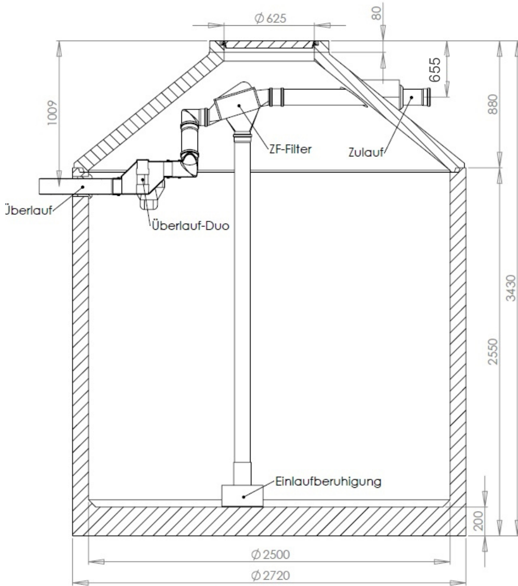
SCHNITT A-A
